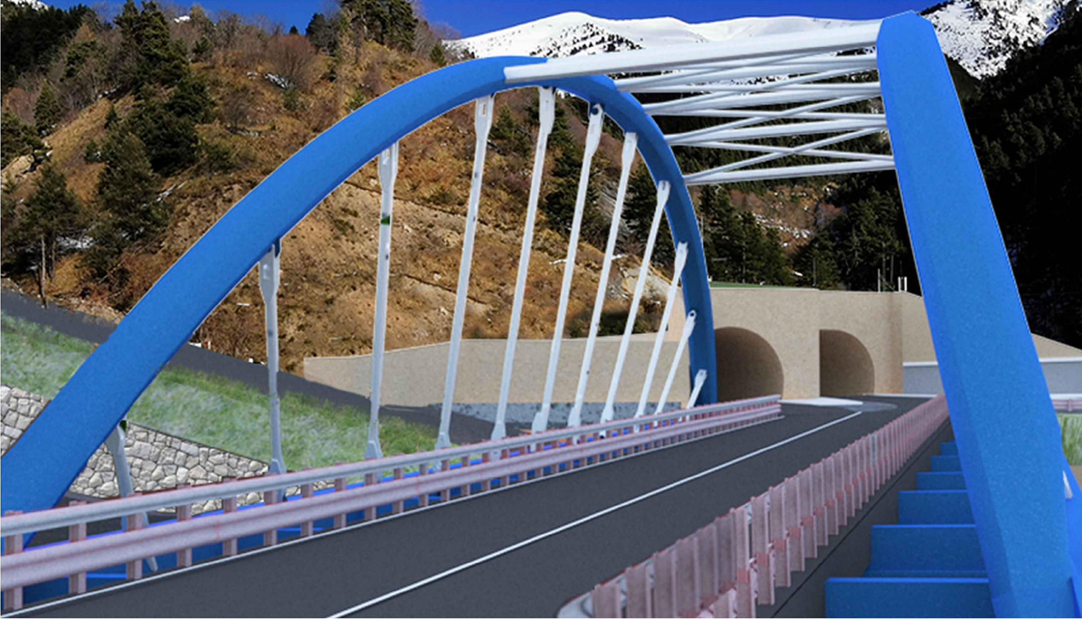
FOTOINSERIMENTO PONTE VALLONE DE LA CA' - SIMULAZIONE CROMATICA IN ACCIAIO CORTEN VERNICIATO SIMILARE ALLA RICOSTRUZIONE DEL PONTE NELLA RD 6204 SIMULATEUR DE PHOTOS DU PONT VALLON DE LA CA' - SIMULATION DE COULEUR SIMILAIRE A RECOSTRUTION DU PONT SUR LA RD 6204
